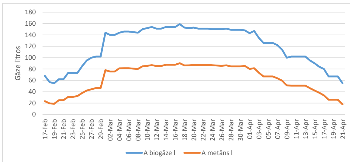
46. attēls. Biogāzes un metāna ieguve no A bioreaktora.
