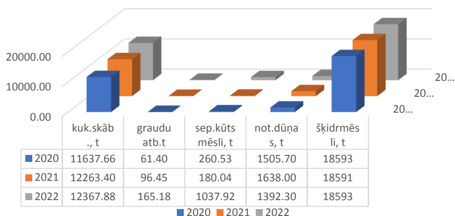
2. att. Izmantotās izejvielas biogāzes stacijā "Ošlejas" kopā pa gadiem, tonnas.
