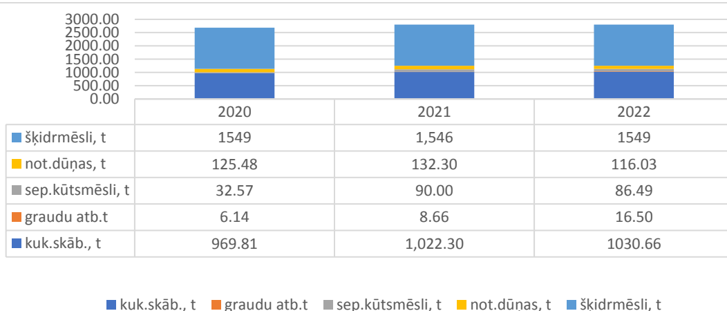
3. att. Izmantotās izejvielas biogāzes stacijā "Ošlejas" vidēji mēnesī un pa gadiem, tonnas.
