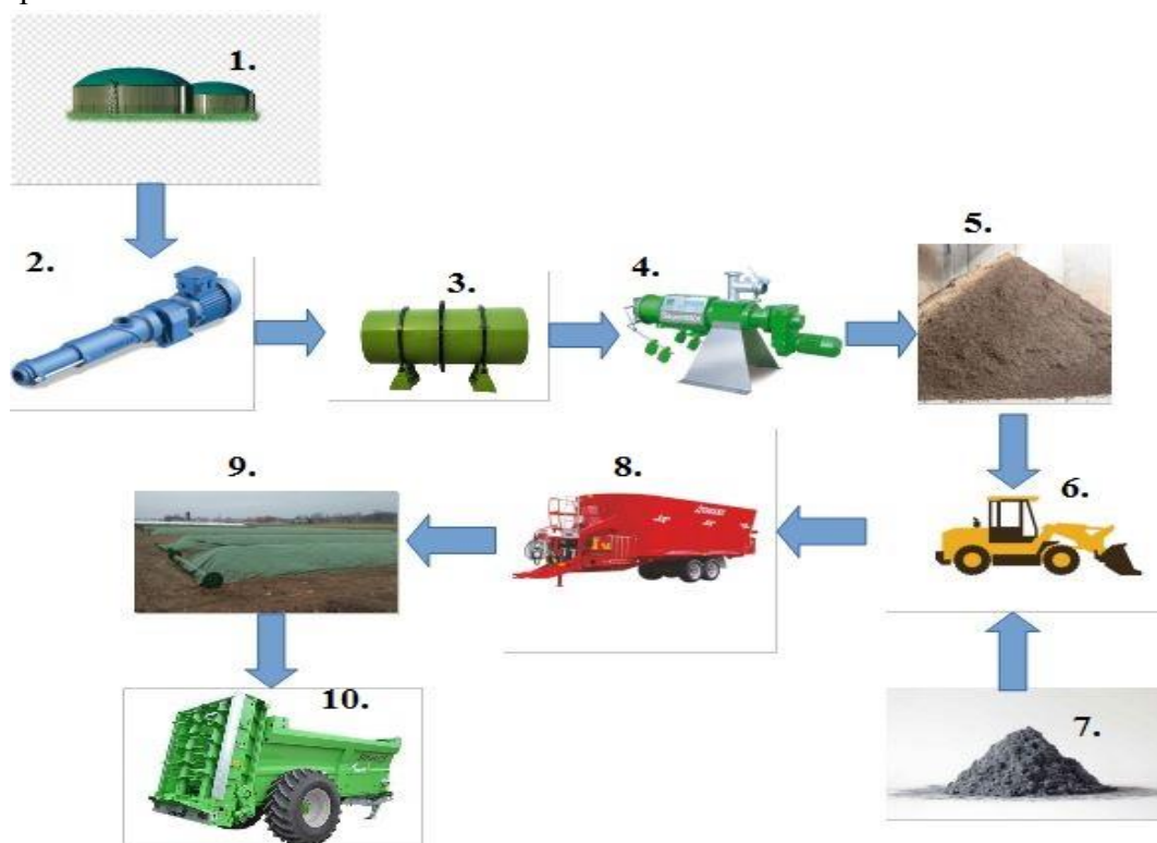
1.4. att. Jaunā mēslojuma sagatavošanas tehnoloģiskā shēma:
