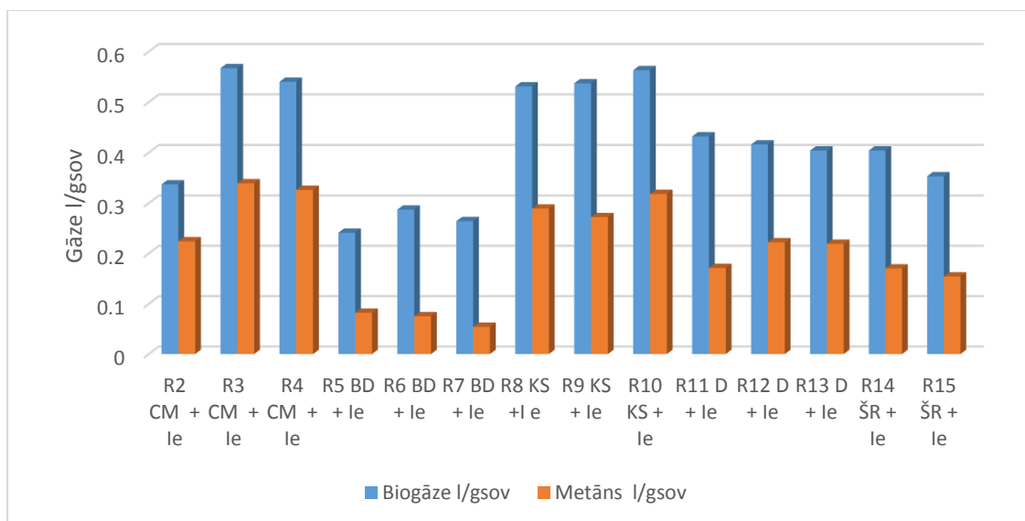
44. attēls. Katrā bioreaktorā saražotais biogāzes un metāna daudzums, L/gsoV.
