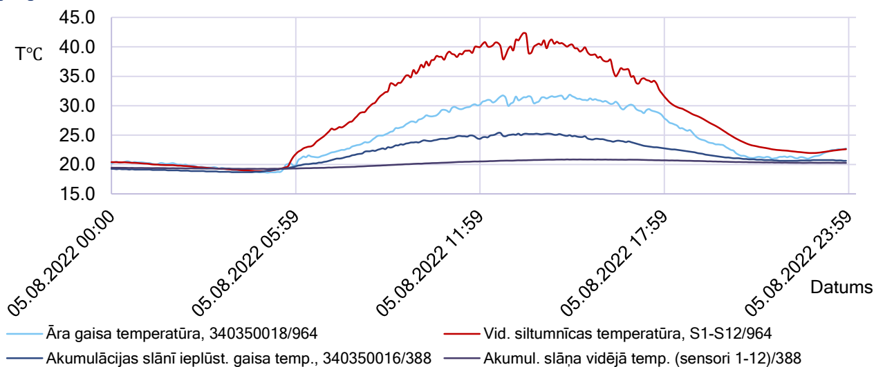
10.5. att. Temperatūra eksperimentālajā siltumnīcā 05.08.2022 zs Skudriņas, T°C
