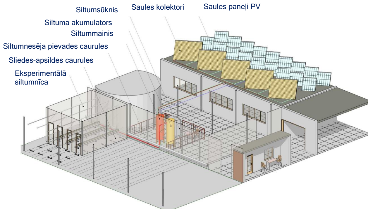
7.1. att. SIA Rītausma eksperimentālās siltumņīcas (50kvm) izstrādes skīču projekts
