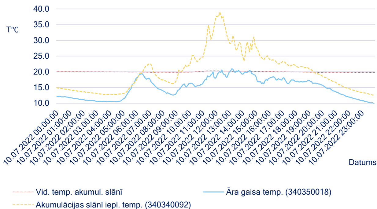
10.1. att. Temperatūras mērījumi eksperimentālajā siltumnīcā 10.07.2022, zs Skudriņas, T°C
