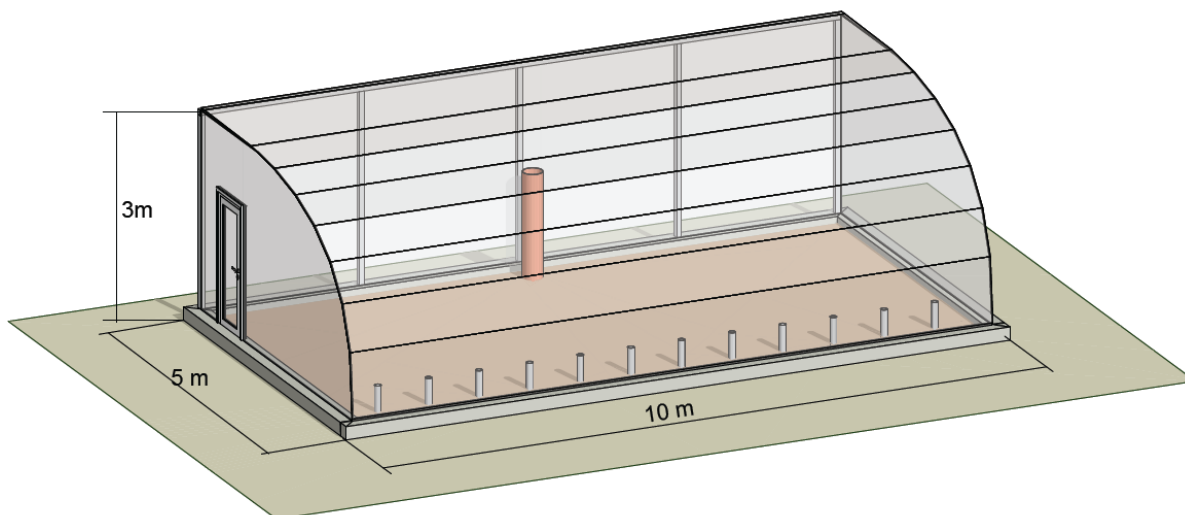
4.6.att. Pasīvās saules enerģijas akumulācijas eksperimentālās siltumnīcas (50kvm) skīču projekts zs “Skudriņas”
