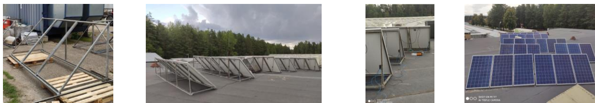
7.8.11. att. Saules elementu montāža uz siltumnīcas jumta
