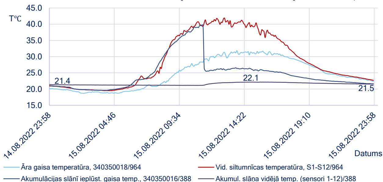
10.6. att. Temperatūra eksperimentālajā siltumnīcā 15.08.2022 zs Skudriņas, T°C
