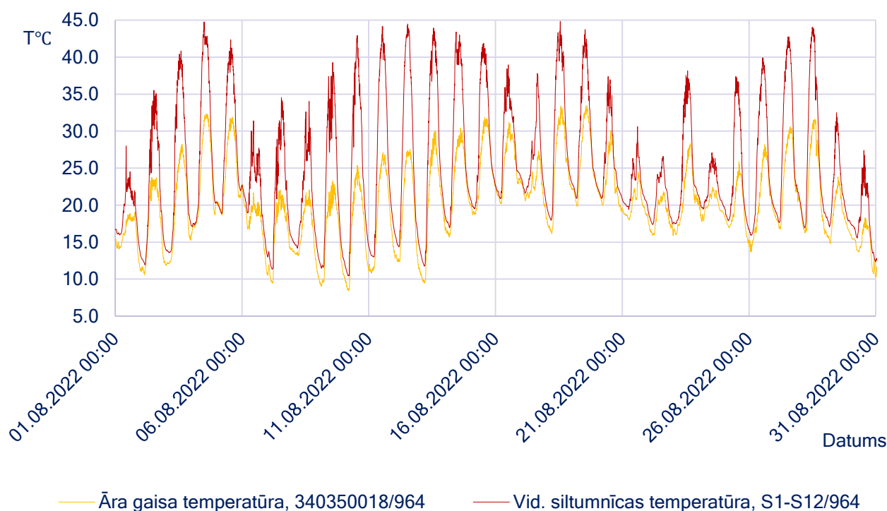
10.2. att. Āra un vidējā iekšējā gaisa temperatūra eksperimentālajā siltumnīcā, 08.2022 zs Skudriņas, T°C
