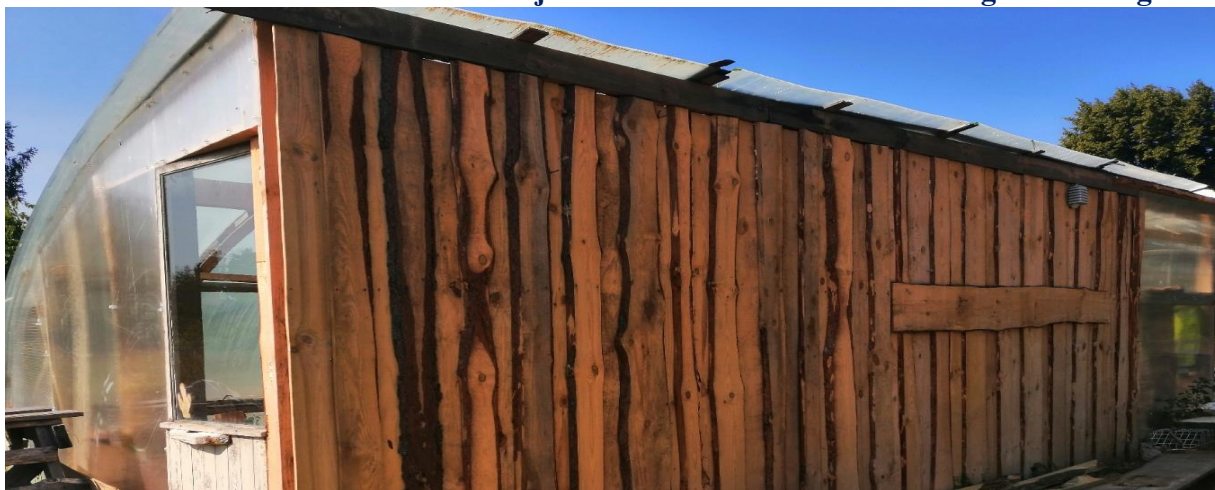
7.2.10. att. Eksperimentālās siltumnīcas ziemeļu puses sienas siltinājums
