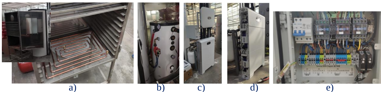
7.8.10. att. Žāvētava a) žāvēšanas spirāle, b) akumulācijas tvertne, c) invertors, d) terminālbloks, e) terminālbloks, skats no iekšienes
