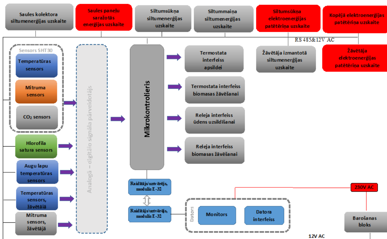
4.1.att. Sensoru un datu uztveršanas sistēmas blokshēma eksperimentālajā siltumnīcā (50kvm) SIA “Rītausma”
