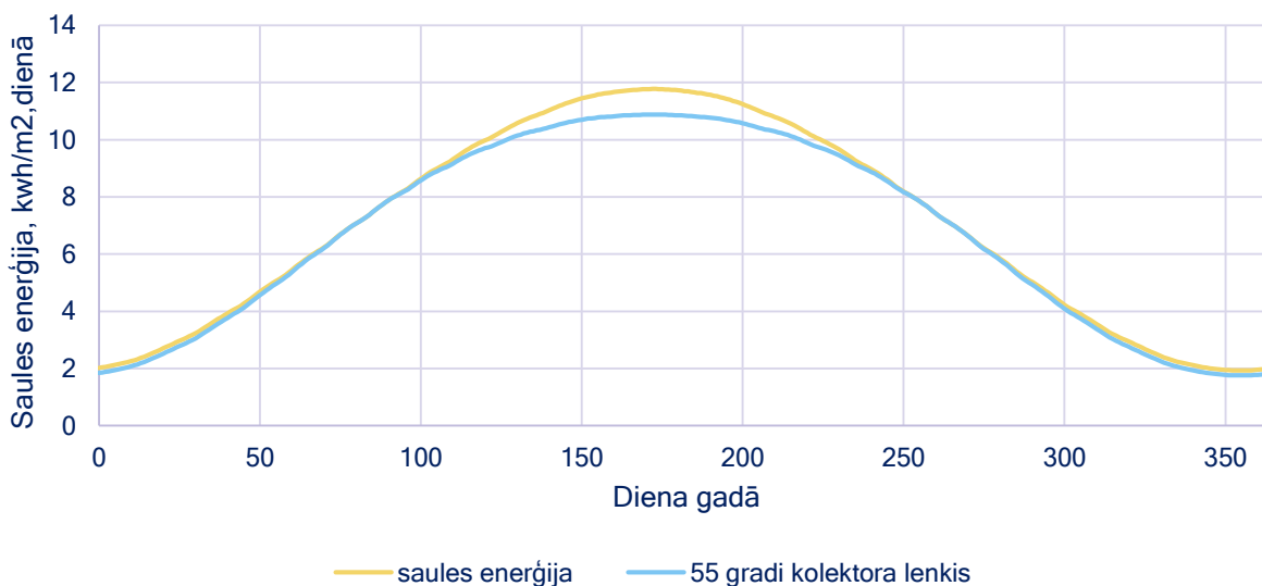
7.4.2. uztvertā Saules enerģija 56° platuma grādā pa dienām
