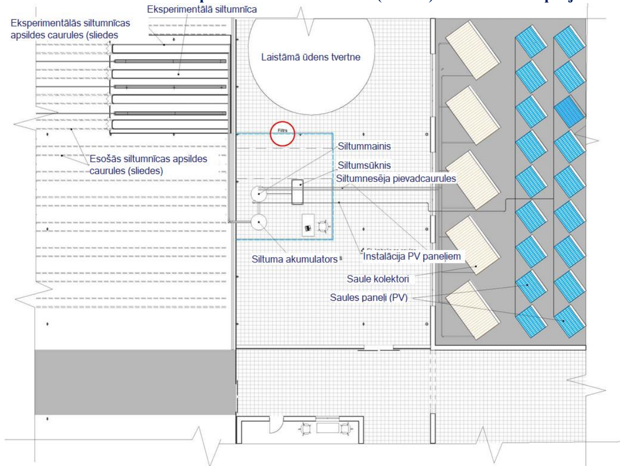
7.2. att. Tehnoloģiskā procesa risinājumu izstrādes skīču projekts, tehnoloģisko iekārtu izvietojums.
