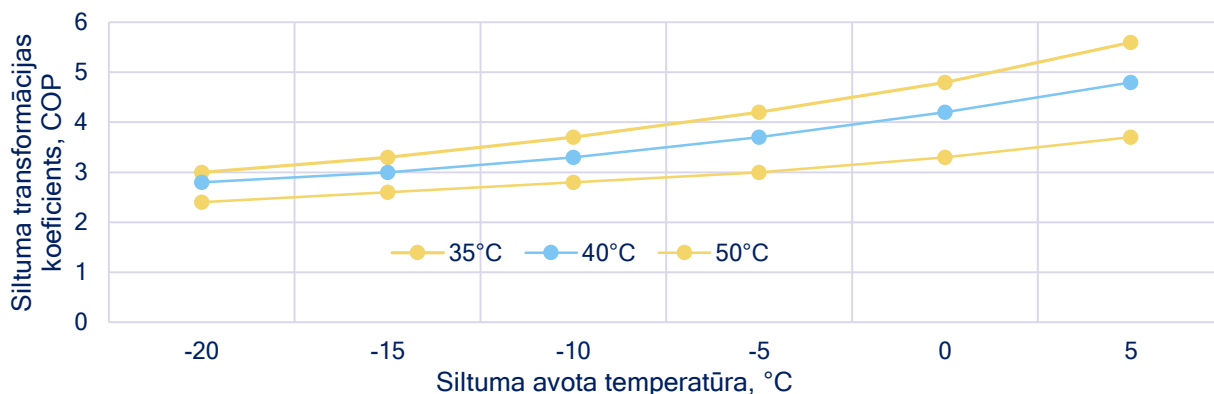
Att. 2.6. Āra gaisa siltuma sūkņu siltuma transformācijas koeficienta COP izmaiņas tendences atkarībā no siltuma avota temperatūras T_a un patēriņam nepieciešamās temperatūras: līdz T_p=35^\circ\text{C} vai līdz T_p=50^\circ\text{C} (pēc dažu ražotāju uzdotiem vidējiem rādītājiem; no literatūras).
