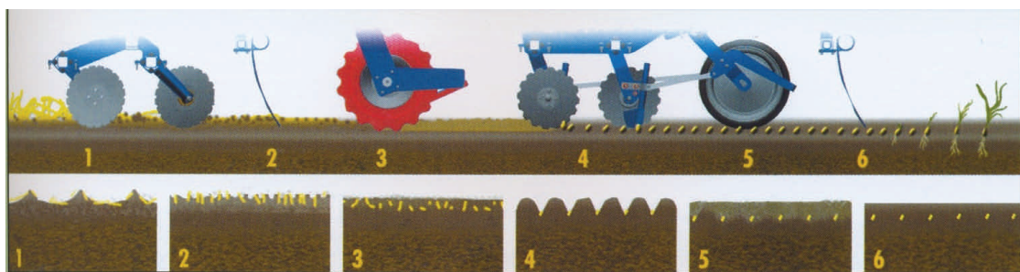
1. att. Minimālā zemes apstrāde un sēja bezaršanas tehnoloģijā: 1 – augsnes lobīšana; 2 – izlīdzināšana; 3 – pieblīvēšana; 4 – graudu iesēšana; 5 – augsnes virskārtas piespiešana; 6 – izlīdzināšana un uzirdināšana.
