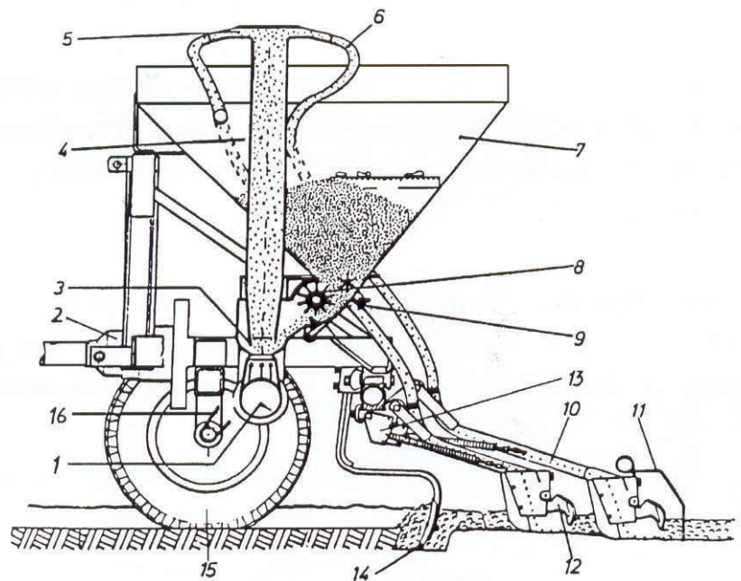
4. att. Pneimatiskās izsējas sējmašīnas darbība.
