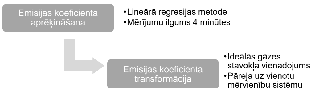
5.6. att. Gāzu koncentrāciju mērījumu transformācijas aprēķina algoritma shematiskais attēlojums.
