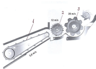
2. att. Kulšanas sistēma ar priekškulēju ( Claas ): 1 – slīpās kameras transportieris; 2 – priekškulējs; 3 – galvenais kuļtrumulis.
