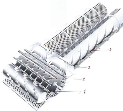
4. att. Rotoru aksiālās plūsmas sistēma (Claas Lexion): 1 – priekškūlējs; 2 – galvenais kuļtrumulis; 3 – atgriežējtrumulis; 4 – labības plūsma.
