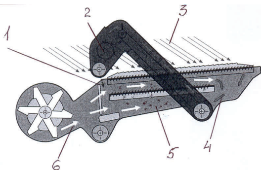
5. att. Pārkuļšanas iekārta (Jeñisej): 1 – Graudi un izkultās vārpas; 2 – kuļtrumulis; 3 – graudu plūsma; 4 – neizkultās vārpas; 5 – tīrie graudi; 6 – vēja plūsma.
