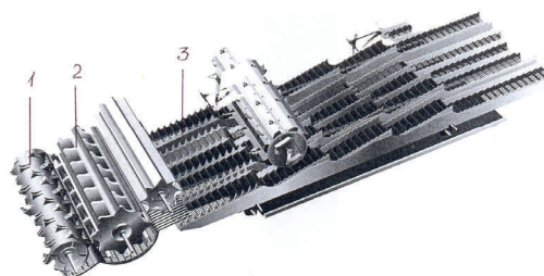
3. att. Graudu atdalīšanas sistēma ar kratītāju ( Claas ): 1 – priekškulējs; 2 – galvenais kuļtrumulis; 3 – salmu kratītājs.
