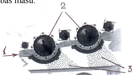
1. att. Divtrumuļu konstrukcija ( Jenisej ): 1 – labības plūsma; 2 – trumuli; 3 – graudu plūsma.
